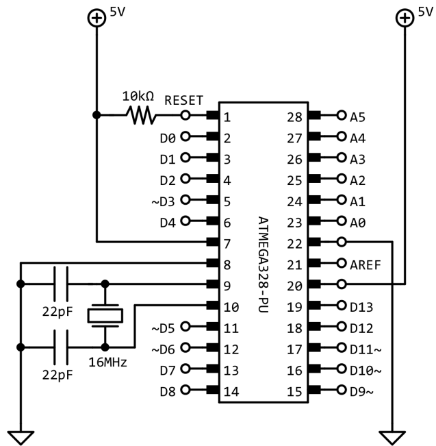
Arduino
