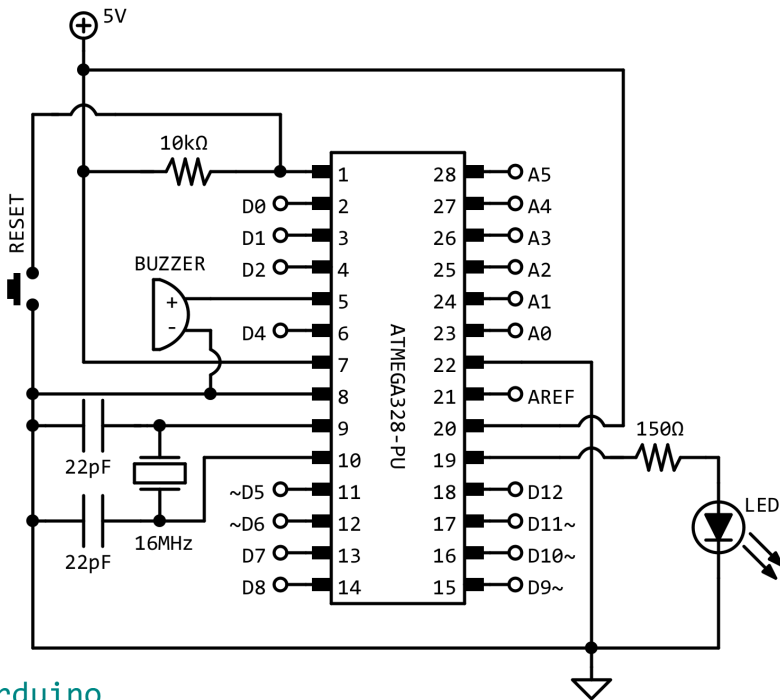
Arduino
